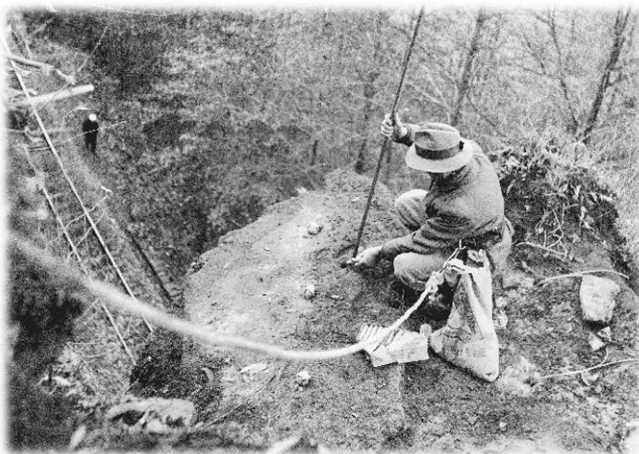
Gründer Karl Gasser beim Laden von Sprenglöchern über dem Trasse der Brünigbahn, 1959
